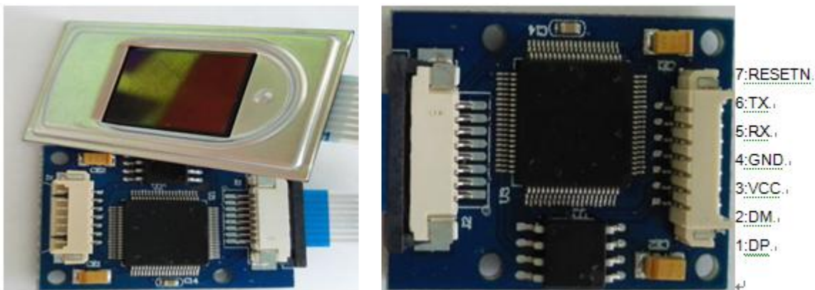
图2-1 SM30指纹识别模块外观图
