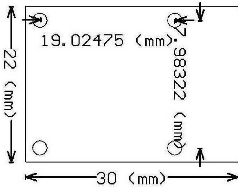
图2-2 SM1S-30主处理板尺寸图
