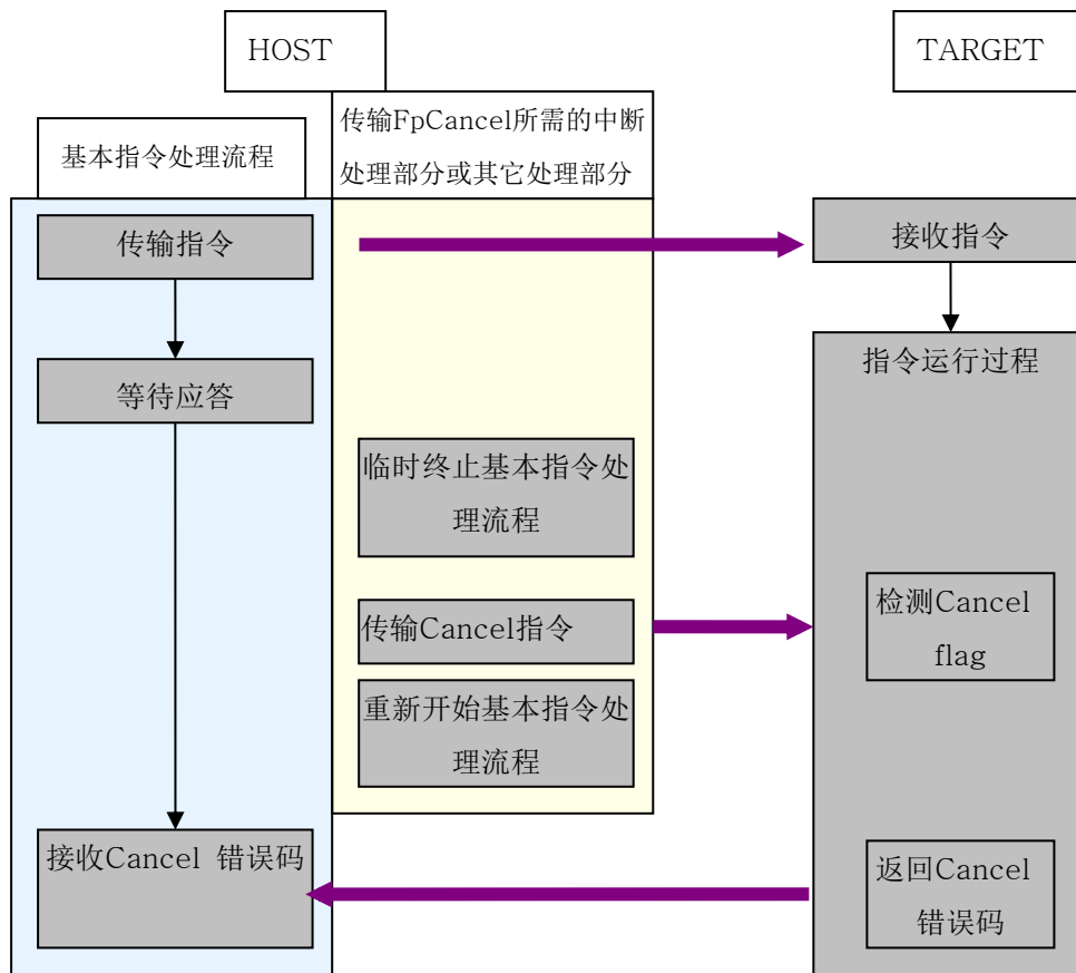
图5-1 FP Cancel过程
