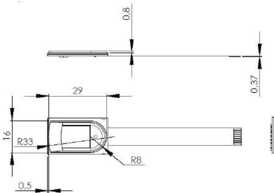
图2-3 FPC1011指纹传感器尺寸图
